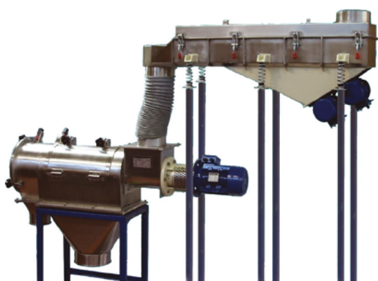
- Gruppo vagliatura/raffinazione
