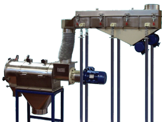
- Gruppo vagliatura/raffinazione
